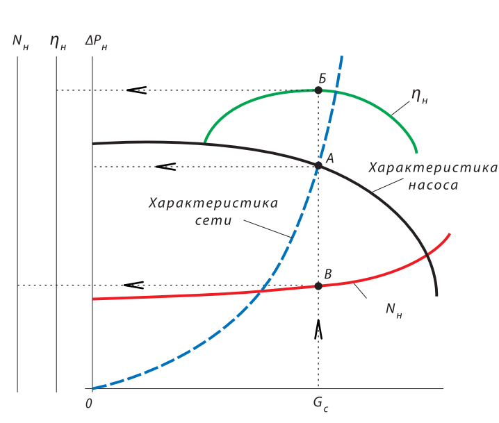
Рис. 11. Характеристика насоса и сети.
