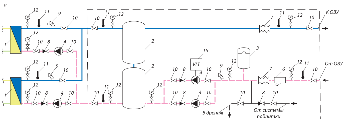
Рис. 10 а. Пример принципиальной схемы гидромодуля с баками-аккумуляторами.
