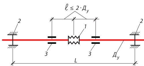
Рис. 13. Установка сильфонного компенсатора торговой марки HYDRA
